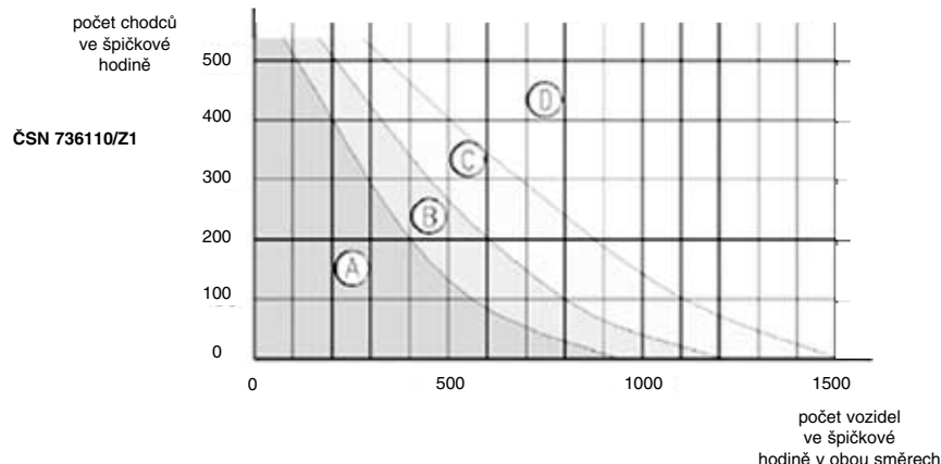
Obrázek 33 – Uplatnění jednotlivých typů opatření pro přecházení chodců v mezikřižovatkových úsecích dvoupruhových místních komunikací s nejvyšší dovolenou rychlostí 50 km/h
